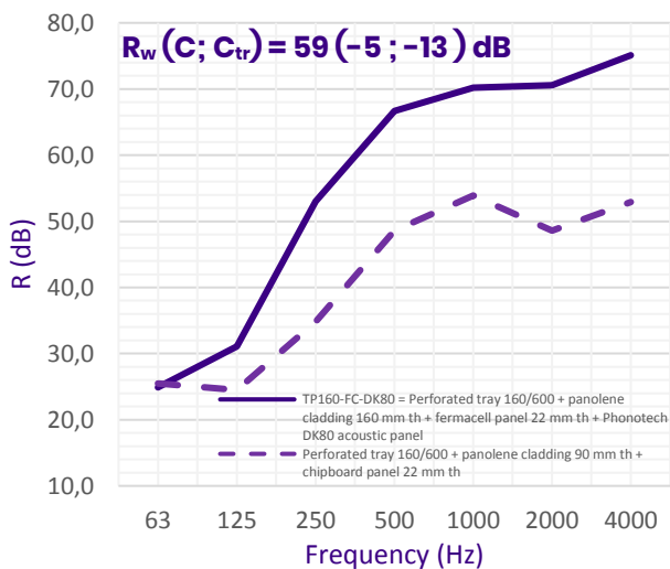
R (dB) per octave band (Hz)
