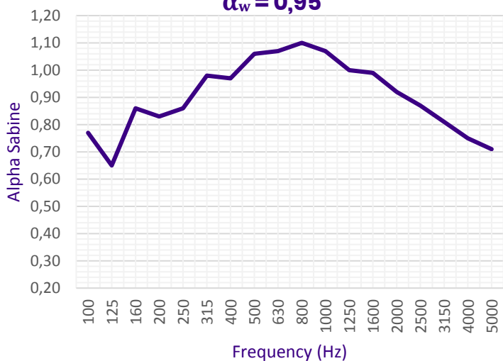
\alpha_p per octave band (Hz)
